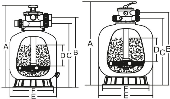
SR-V350-15 ~ SR-V700-15
